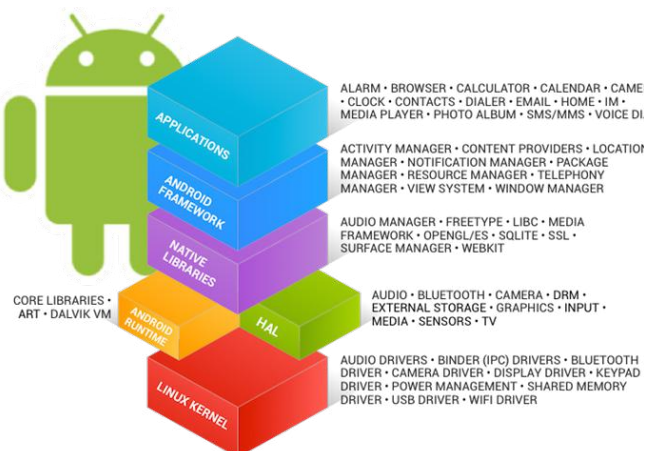
Représentation de la pile Android
